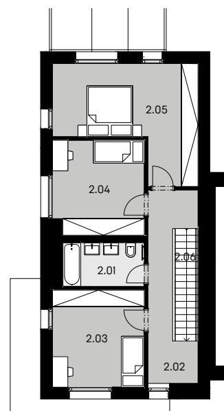
2.NP
