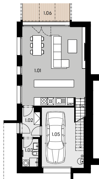
1.NP
